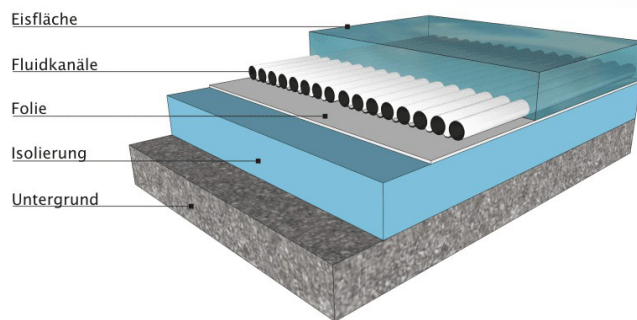
Abbildung 16: Aufbau Eisfläche
